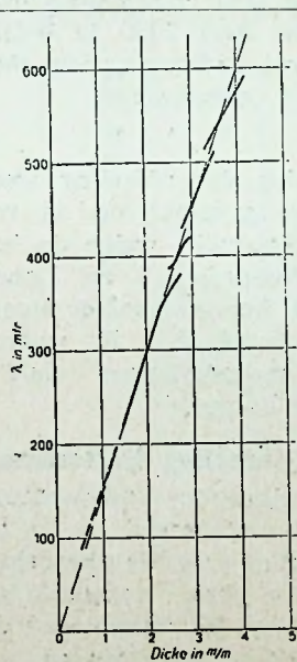
Fig. 2. Medesleepingsverschijnselen evenals bij gekoppelde kringen, ontstaande door wisselwerkingen tusschen diktetrilling en lengtetrilling.
