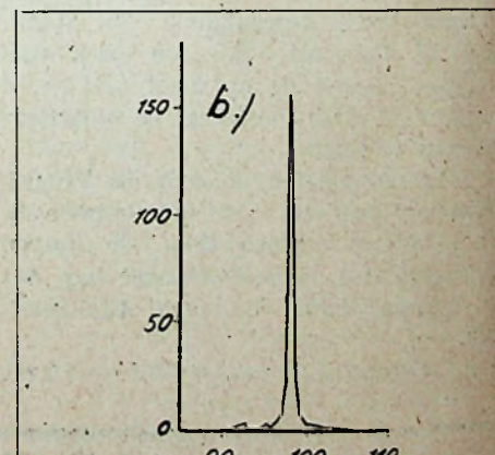
Fig. 3. Resonantie-curve van hetzelfde kwartsplaatje als in fig. 1 bedoeld, bij gelijke dikte, maar tot één frequentie teruggebracht.
