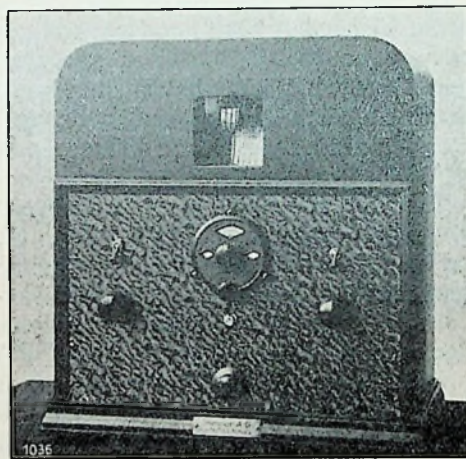
Groote Televisie-ontvanger der Telehor A.G. met ingebouwd lampgenerator en schakelaar voor overgang van luidspreker-ontvangst op televisie-ontvangst; het apparaat bezit regelingen voor de synchronische frequentie, de sterkte der signaal-stroom, den motorstroom en de beeld-phase. Verder een hoofdschakelaar.
