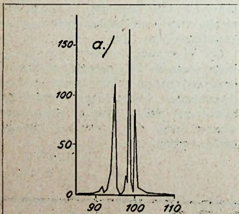
Fig. 1. Resonantie-curve van een kwartsplaatje, dat in meer dan één frequentie genereert.
