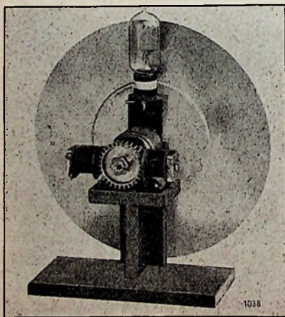
Schijf met glimlamp, aandrijfmotor en toonrad van de Deutsche Fernseh Gesellschaft. Het beeld wordt aan de andere zijde van de schijf door een beeldvenster en vergrootglas bekeken.
