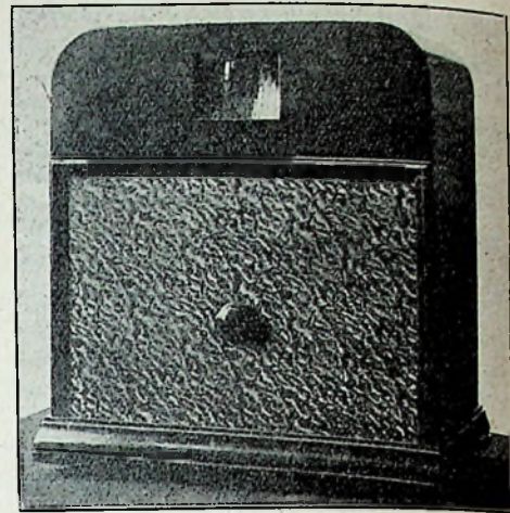
Kleine televisie-ontvanger, die de frequentie van het wisselstroomlichtnet voor de synchronisatie gebruikt. In het midden bevindt zich de knop voor de phase-regeling.
